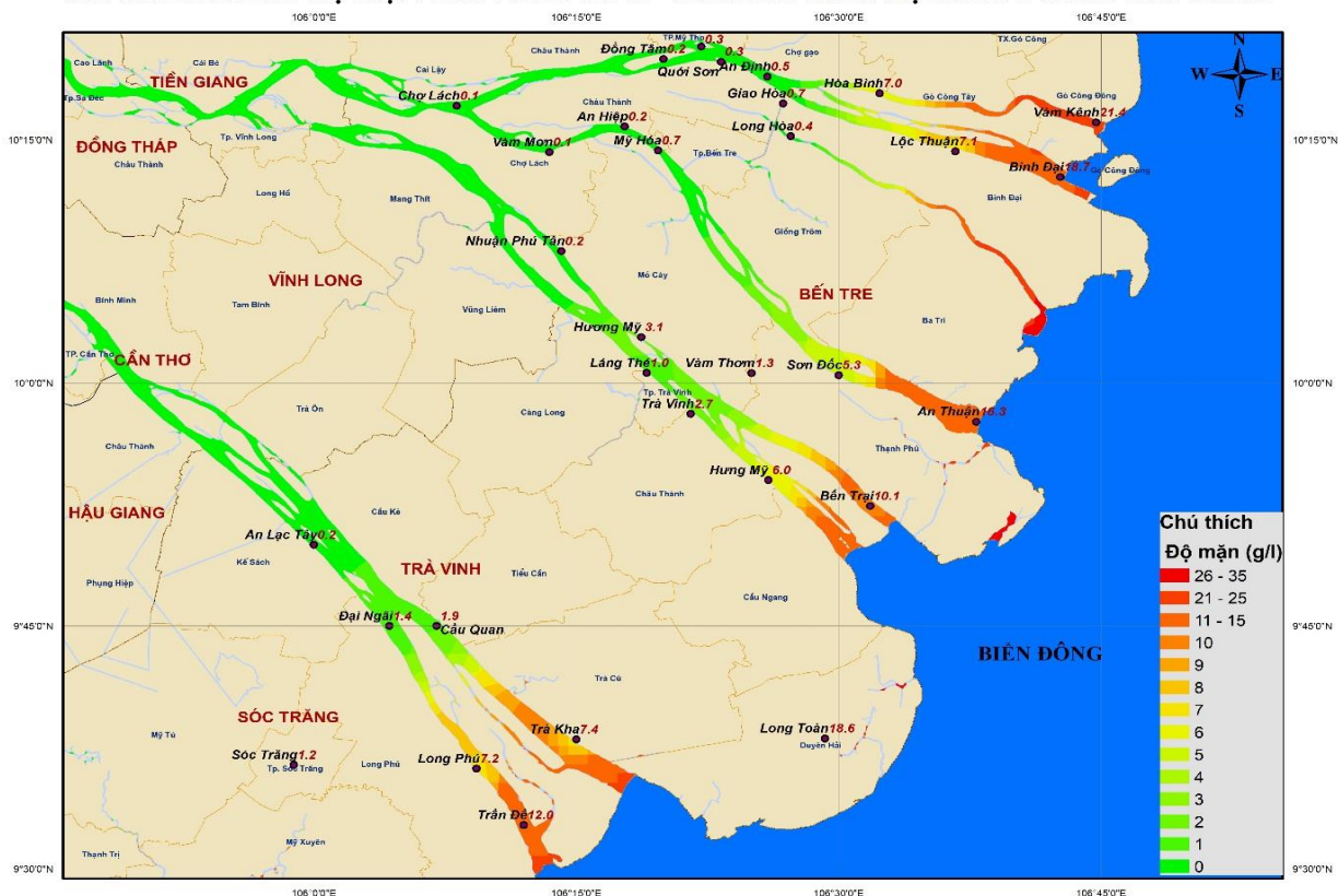
BẢN ĐỒ PHÂN BỐ ĐỘ MẶN CAO NHẤT TỪ 11 - 20/05/2021 TRÊN HỆ THỐNG SÔNG CỬU LONG
