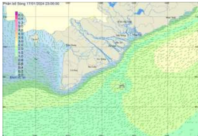
Hình 2: Bản đồ sóng dự báo lúc 23h00 ngày 17/01
