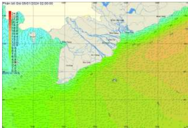
Hình 1: Bản đồ gió dự báo lúc 02h ngày 05/01
