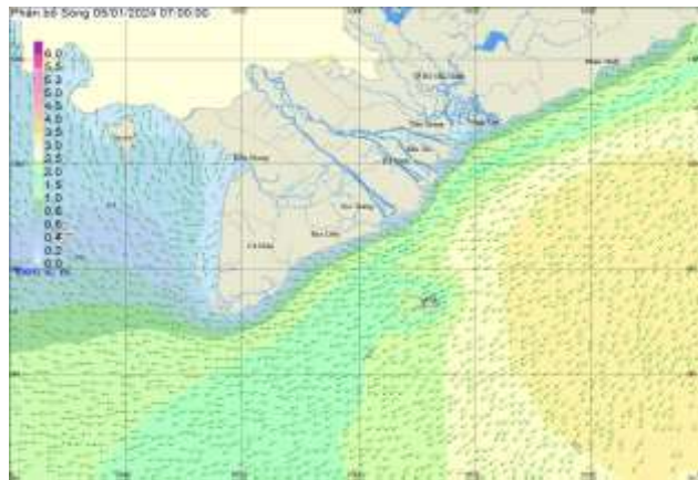
Hình 2: Bản đồ sóng dự báo lúc 07h ngày 05/01
