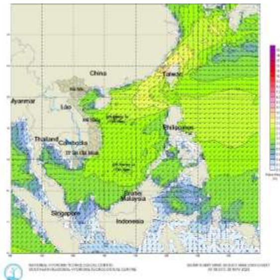
Hình 2. Bản đồ dự báo sóng lúc 13h ngày 30/11/2023
