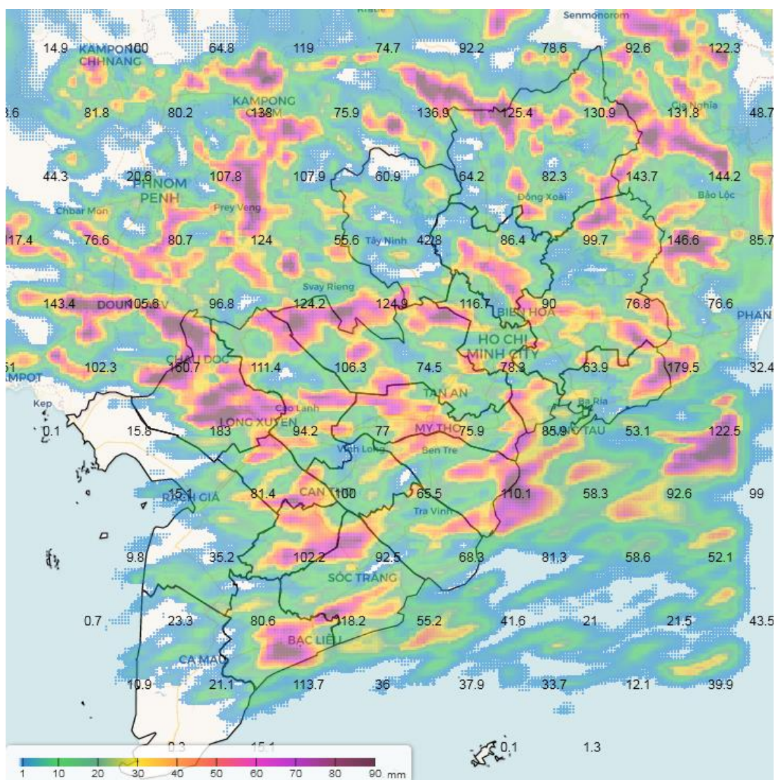
Bản đồ dự báo mưa từ 01h ngày 15/10 đến 01h ngày 16/10 ở khu vực Nam Bộ
