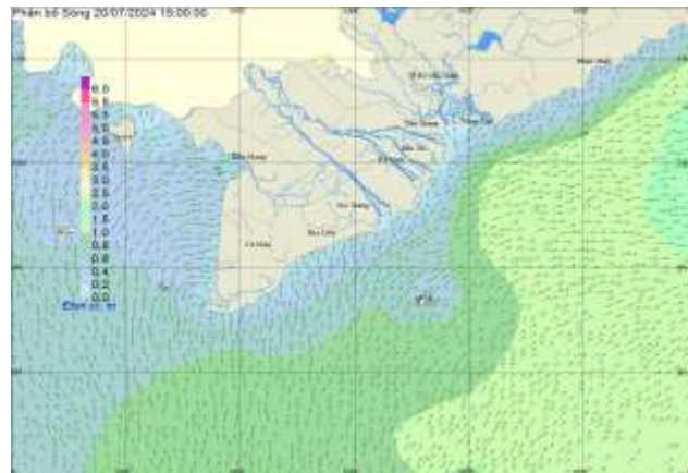
Hình 2: Bản đồ sóng dự báo lúc 15h00 ngày 20/07
