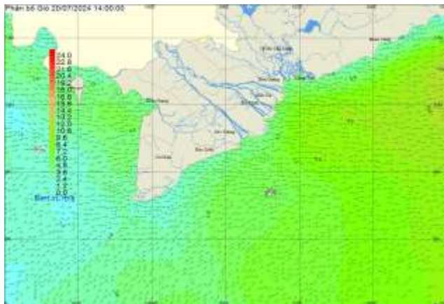
Hình 1: Bản đồ gió dự báo lúc 14h00 ngày 20/07
