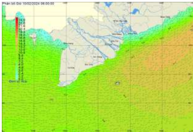
Hình 1: Bản đồ gió dự báo lúc 06h00 ngày 10/02
